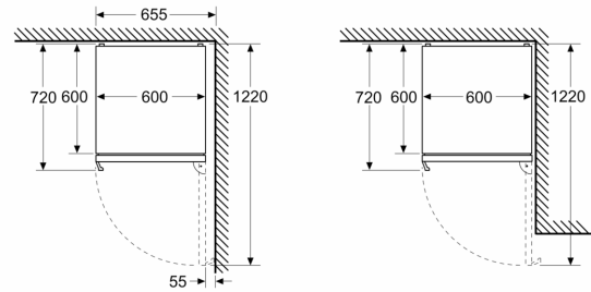
Matmenys, mm
