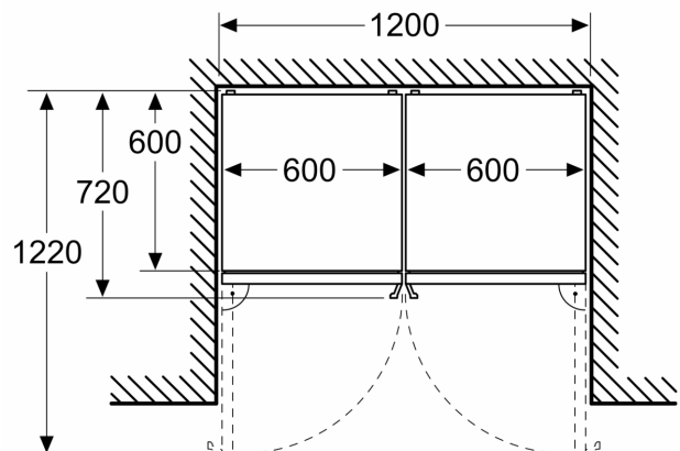
Matmenys, mm
