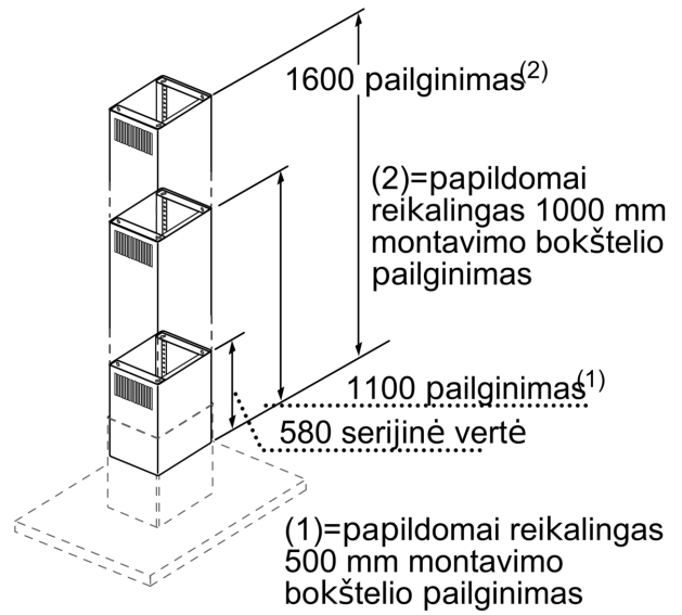
Matmenys mm
