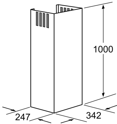
Matmenys mm
