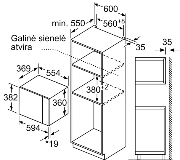
Matmenys, mm
