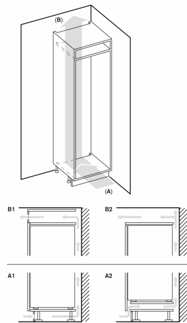
A: Ingresso aria \geq 200 \text{ cm}^2 ; opzioni ventilazione A1 o A2 B: Uscita aria \geq 200 \text{ cm}^2 ; opzioni ventilazione B1 o B2
