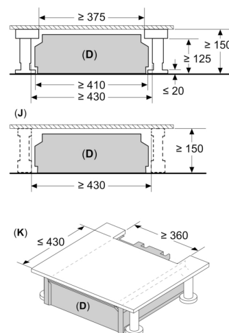
Dimensioni in mm Vista frontale
