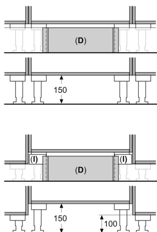
Dimensioni in mm Varianti zoccoli per modulo robot
