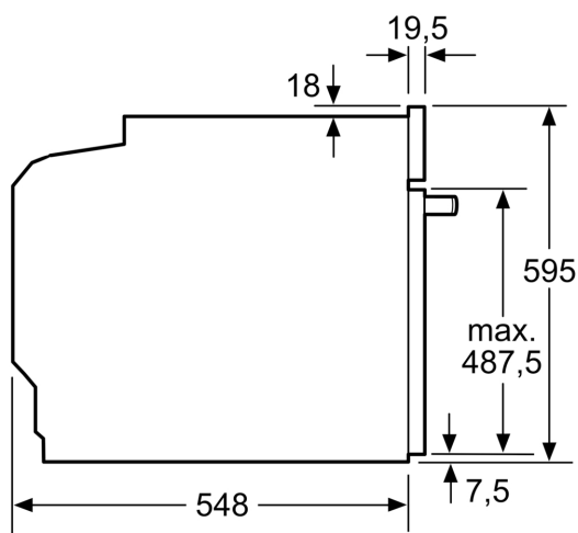
Méretek mm-ben
