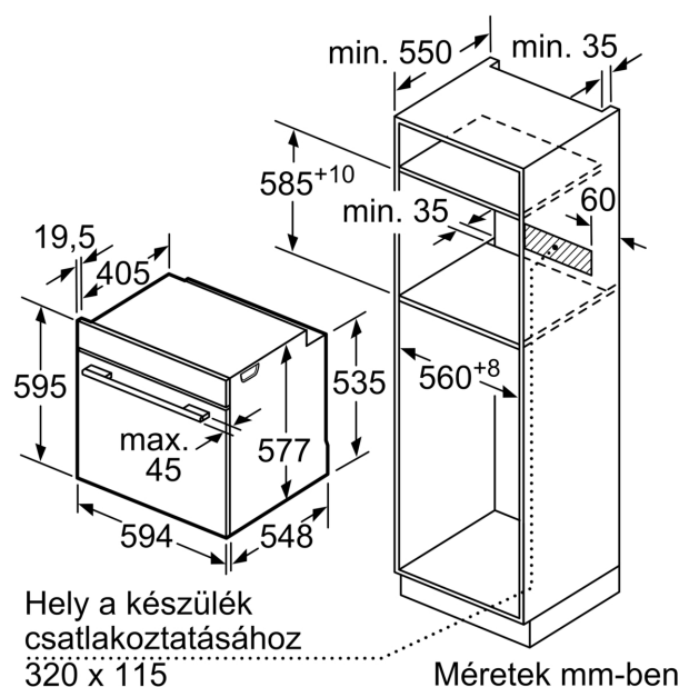
Méretek mm-ben
