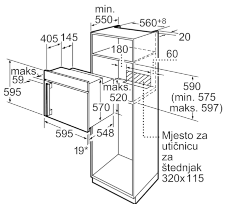
* Kod metalnih pročelja 20mm mjere u mm
