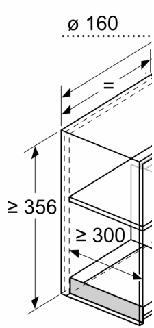
mjere u mm Primjer ugradnj
