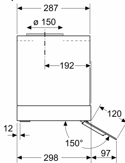
Mjere u mm Bočni prikaz
