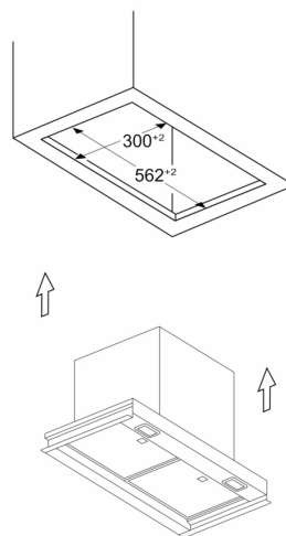
Mjere u mm Primjer ugradnje u urezu namještaja
