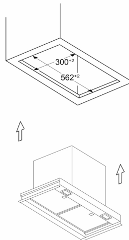
Mjere u mm Primjer ugradnje u urezu namještaja
