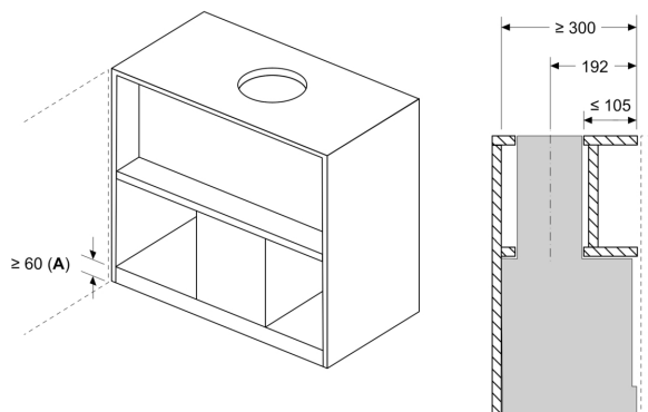
Mjere u mm Primjer ugradnje s policom za začine
