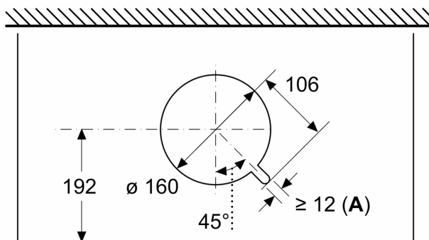
Mjere u mm Prikaz odozgo
