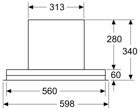
Mjere u mm Pogled sprijeda
