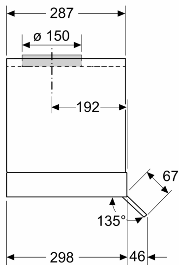
Mjere u mm Bočni prikaz
