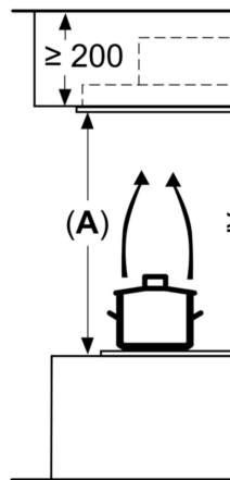
Mesures en mm Évacuation d'air
