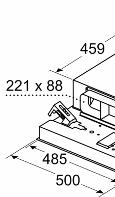
Mesures en mm
