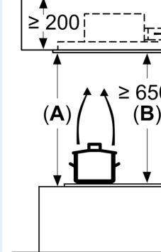
Mesures en mm Circulation d'air
