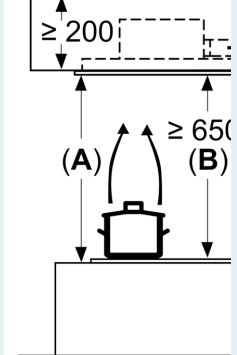
Mesures en mm Circulation d'air
