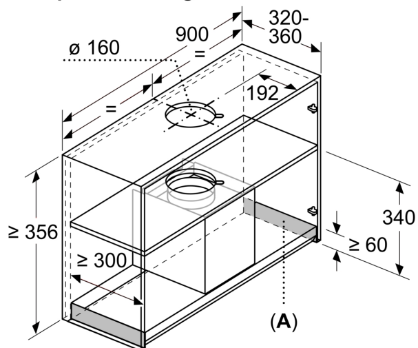
Mesures en mm Exemple de montage
