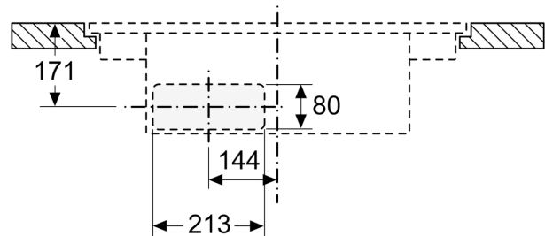
Mesures en mm Vue avant – découpage de l'unité pour la recirculation libre
