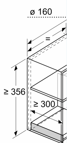
mesures en mm Exemple de montage
