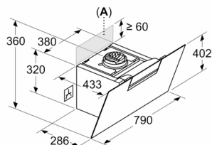
Mesures en mm Appareil en mode circulation d'air sans conduit
