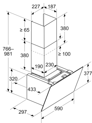
Mesures en mm Appareil en mode d'évacuation d'air
