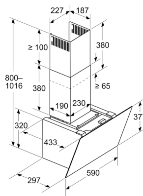
Mesures en mm Appareil en mode circulation d'air
