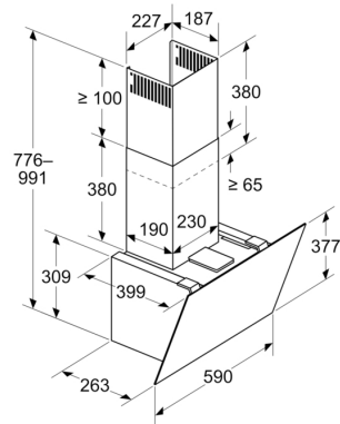
Mesures en mm Appareil en mode circulation d'air
