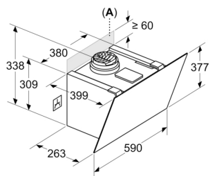
Mesures en mm Appareil en mode circulation d'air sans conduit
