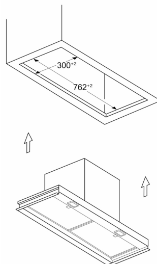
Mesures en mm Exemple d'installation dans une découpe de meuble
