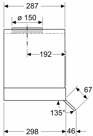
Mesures en mm Vue latérale
