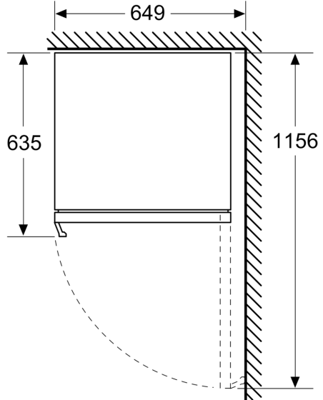
Mitat mm
