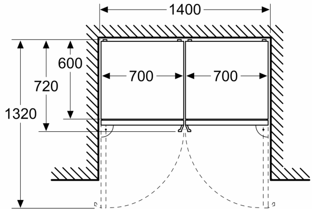
Mitat mm
