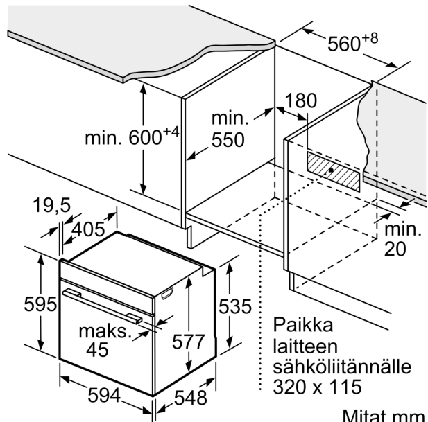
Mitat mm
