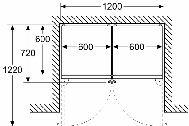
Mõõdud (mm)
