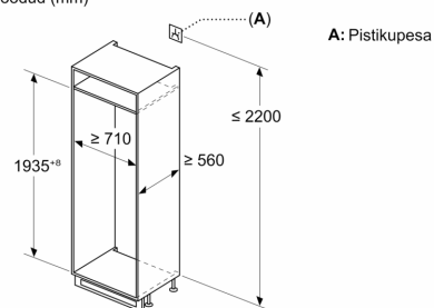
Mõõdud (mm)
