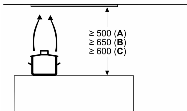
Mõõdud (mm)
