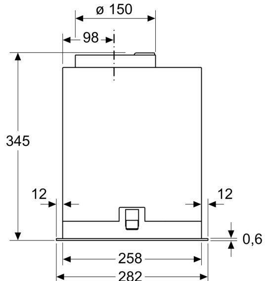
Mõõdud (mm)
