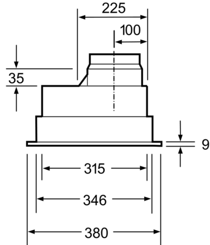
Mõõdud (mm)
