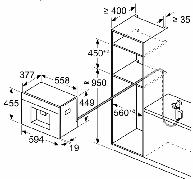
Mõõdud (mm)
