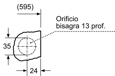
Detalle Z
