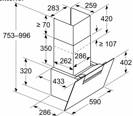
Dimensiones en mm Aparato en modo de salida de aire al exterior
