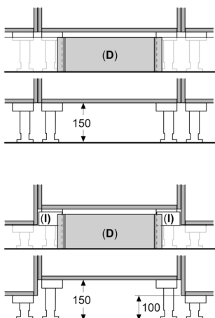
Dimensiones en mm Variantes de zócalo para módulo del robot
