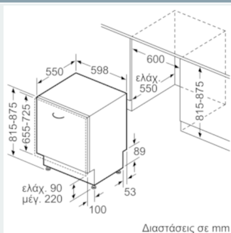
Σχέδια διαστάσεων
