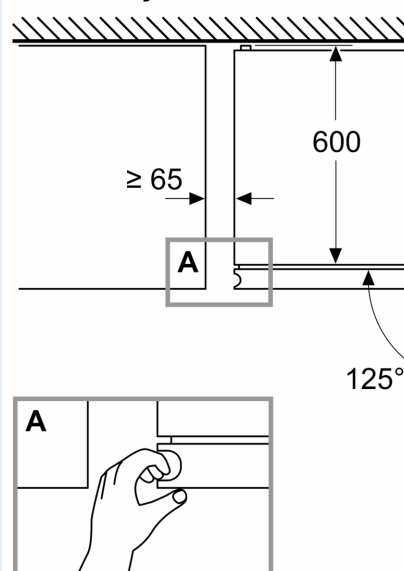
Διαστάσεις σε mm
