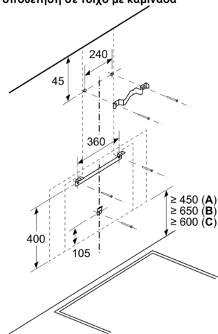
Διαστάσεις σε mm Τοποθέτηση σε τοίχο με καμινάδα
