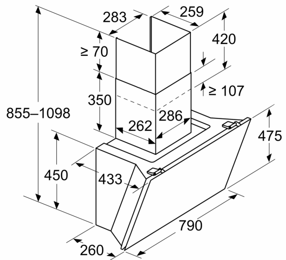
Διαστάσεις σε mm Συσκευή σε λειτουργία εξαερισμού
