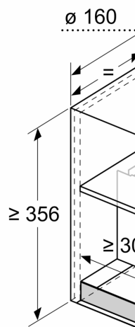
Maße in mm Einbaubeispiel
