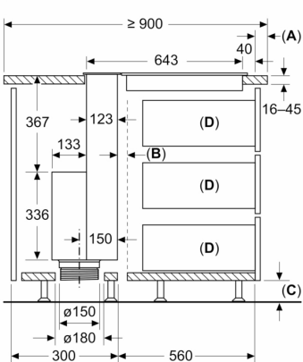
Maße in mm Nahtloser, aufgesetzter Einbau (Sonderzubehör erforderlich)
