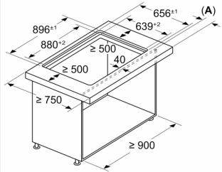
Maße in mm Kombination mit Elektrokochfeld Nahtloser, flächenbündiger Einbau
