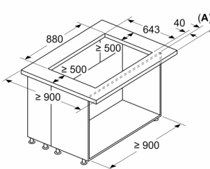
Maße in mm Kombination mit Elektrokochfeld Nahtloser, aufgesetzter Einbau
