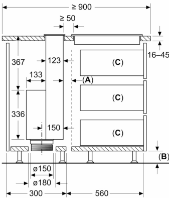
Maße in mm Standard, aufgesetzter Einbau
