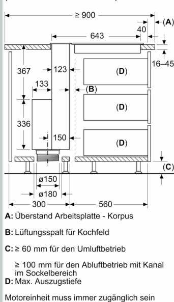
Maße in mm Nahtloser, aufgesetzter Einbau (Sonderzubehör erforderlich)
