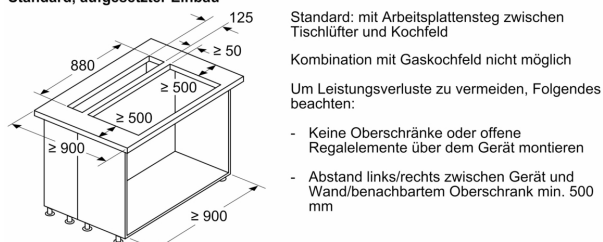
Maße in mm Kombination mit Elektrokochofeld Standard, aufgesetzter Einbau
