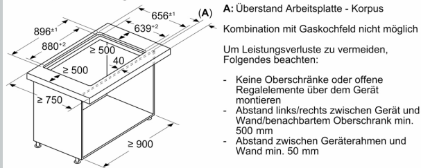
Maße in mm Kombination mit Elektrokochofeld Nahtloser, flächenbündiger Einbau
