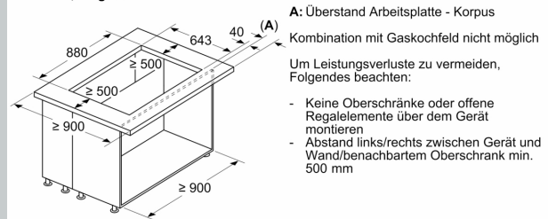
Maße in mm Kombination mit Elektrokochofeld Nahtloser, aufgesetzter Einbau
