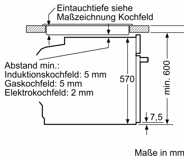
Einbau mit einem Kochfeld.
