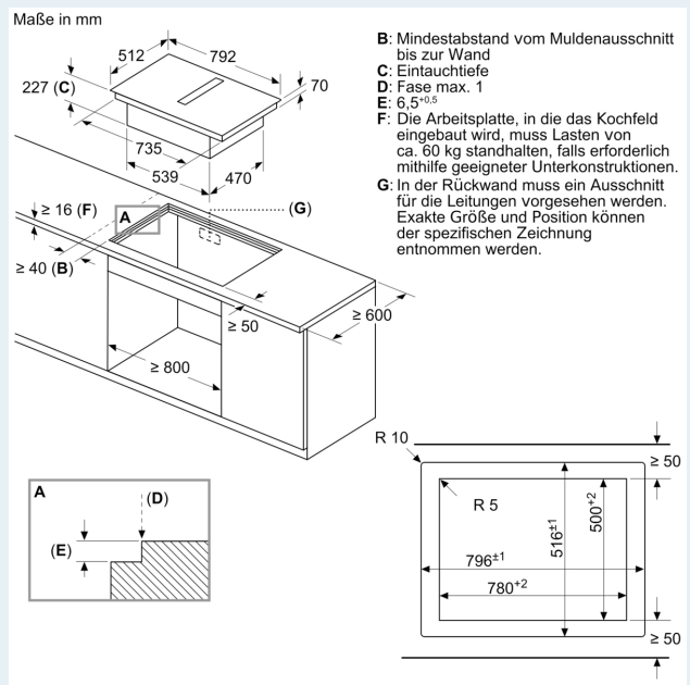
Maße in mm Vorderansicht – Geräteausschnitt für ungefasste Umluft
