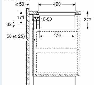
Maße in mm Seitenansicht
