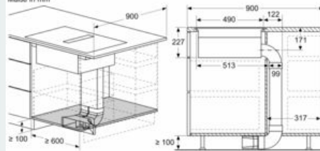
A: 90° Bogen Größe S B: Verbindungsmanschetten C: Gerades Rohr Maße in mm
