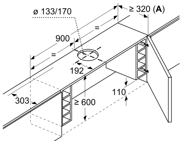
Maße in mm Montage Flachschirmhaube mit Absenkrahmen
