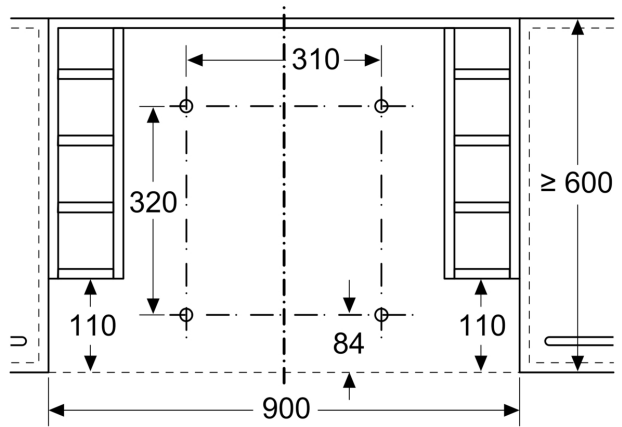
Montage Flachschildhülle mit Absenkrahmen Möbel mit seitlichen Regalfächern Montage direkt an der Küchenwand
