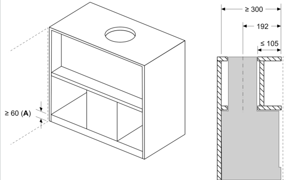
Maße in mm Einbaubeispiel mit Gewürzregal
