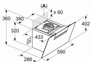
Maße in mm Gerät im Umluftbetrieb ohne Abluftkanal
