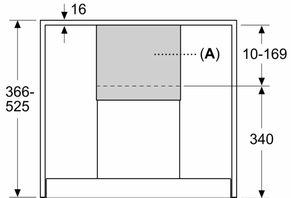
Maße in mm Einbaubeispiel für Schrankhöhe 366-525 mm
