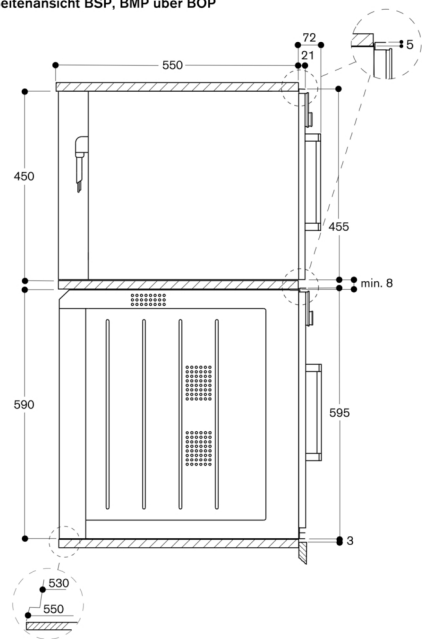
Seitenansicht BSP, BMP über BOP
