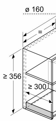
Maße in mm Einbaubeispiel
