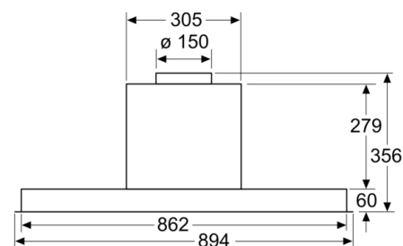
Masse in mm Frontansicht
