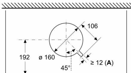
A: Kabledurchführung
