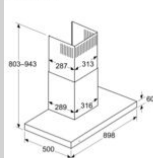
Ansicht Umluft
