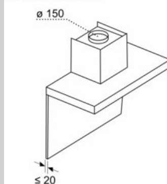
Wandblendentiefe
