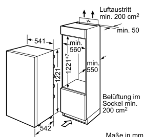
Maße in mm Empfehlung Spaltmaße für Flachscharnier
